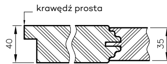
Przekrój poziomy drzwi Nestor
