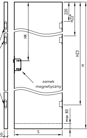
Skrzydła bezprzylgowe rozwiernie Standard 10, Modern, Plus
