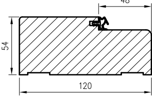
Przekrój ościeżnicy drewnianej do drzwi OLIMP EI60
