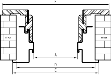
Profil ościeżnicy
