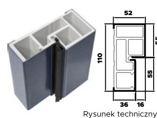
Ościeżnica symetryczna Optimum
