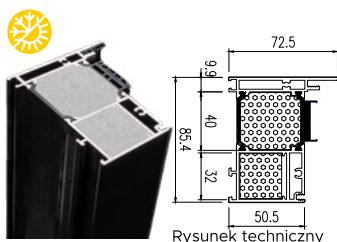
Rysunek techniczny
