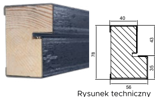
Ościeżnica Stalowo- drewniana Basic 3.0
