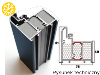
Ościeżnica Alumiiniowo- drewniana Plus
