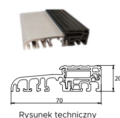
Rysunek techniczny
