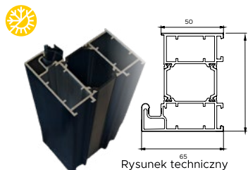
Rysunek techniczny
