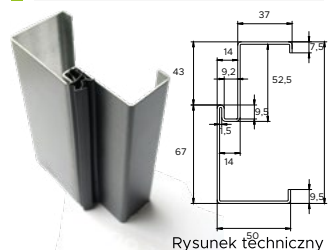
Przekrój łącznika kątowne- go Termo 90°
