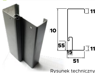
Rysunek techniczny
