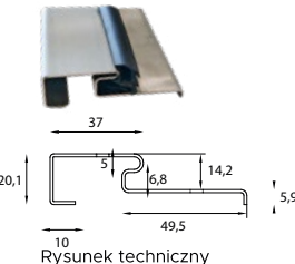
Rysunek techniczny
