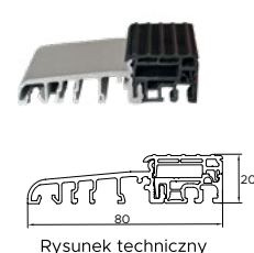
Rysunek techniczny
