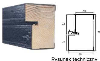
Rysunek techniczny
