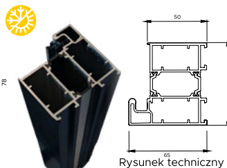
Ościeżnica symetryczna Prima
