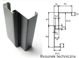
Ościeżnica Alu Hybrid
